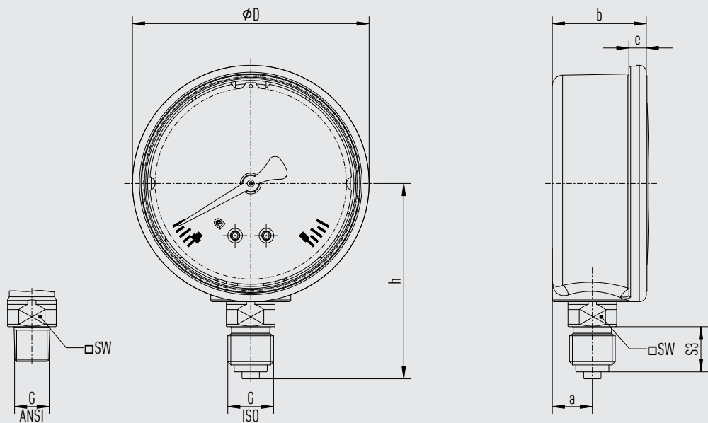
Typ 113.13, Anschluss radial unten
