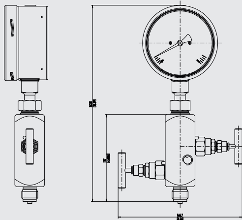
Mit Ventil-Typ IV20
