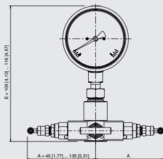
Mit Ventil-Typ IVM
