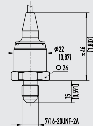
Mit Kabelausgang
