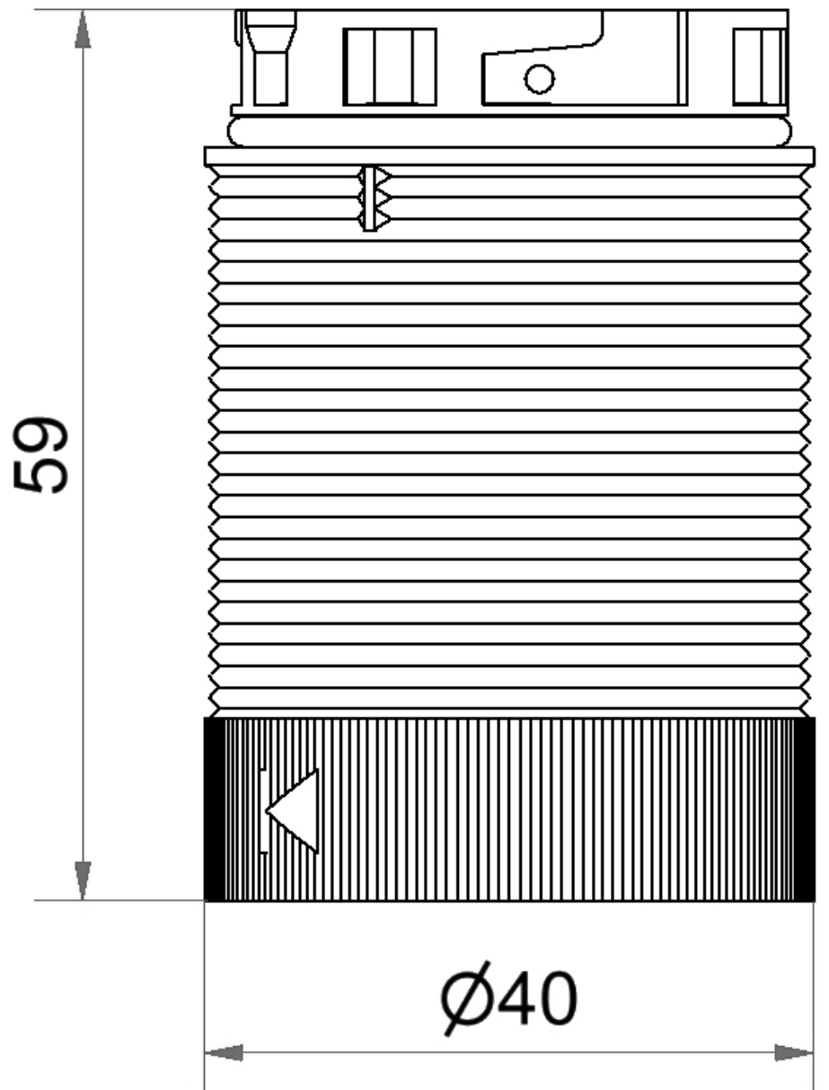
MASSZEICHNUNG
