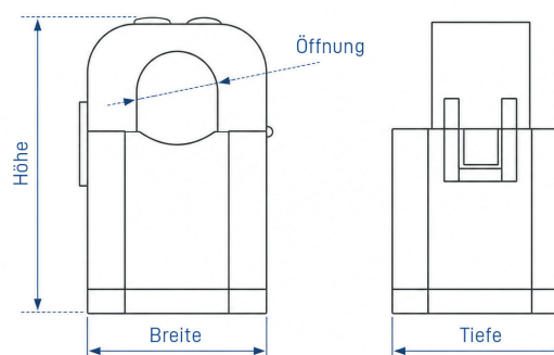
Abmessung Klappstromwandler VEM103-CT 63
