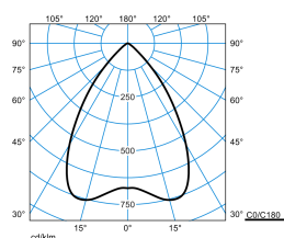
InperlaL G2 C07 HR19 2700-840 01 + RG-PC
