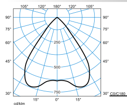
InperlaL G2 C07 HR19 2700-840 ETDD 01
