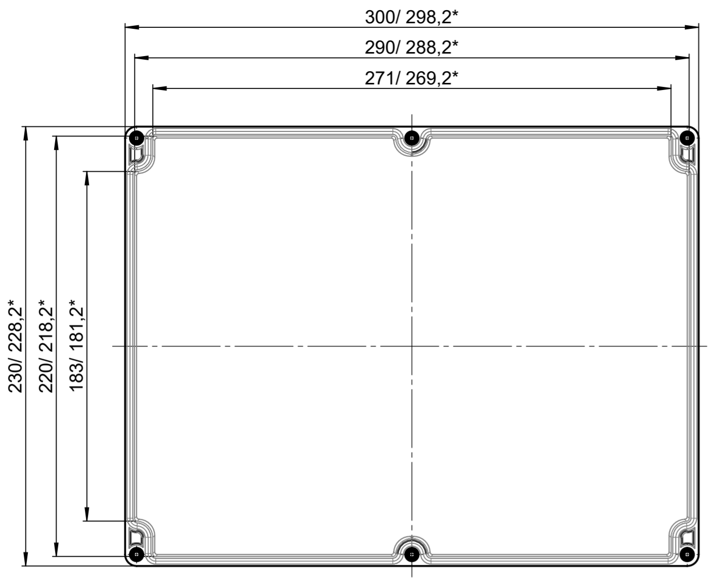
Deckel / Lid
