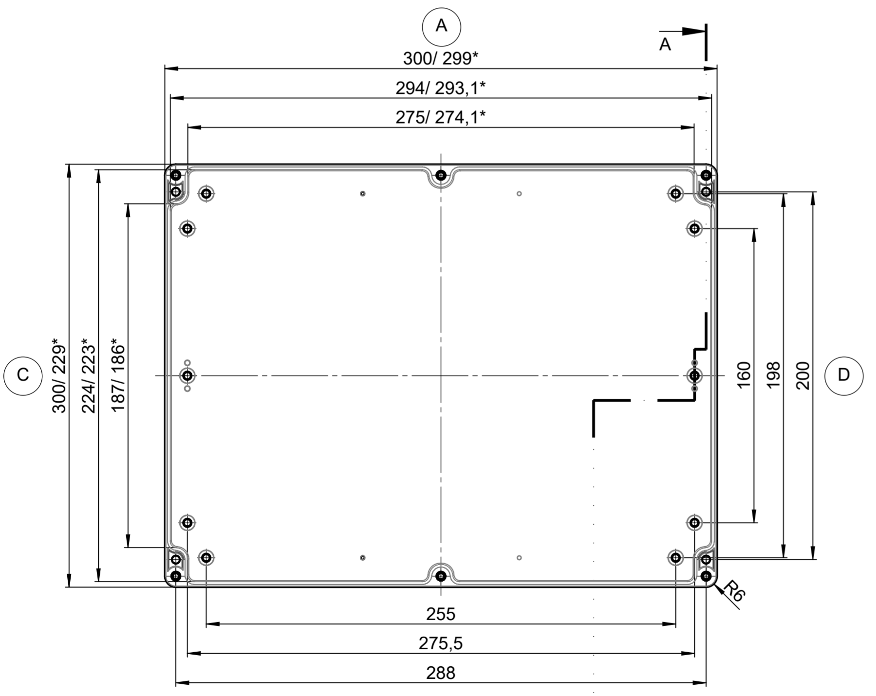
Unterteil / Base
