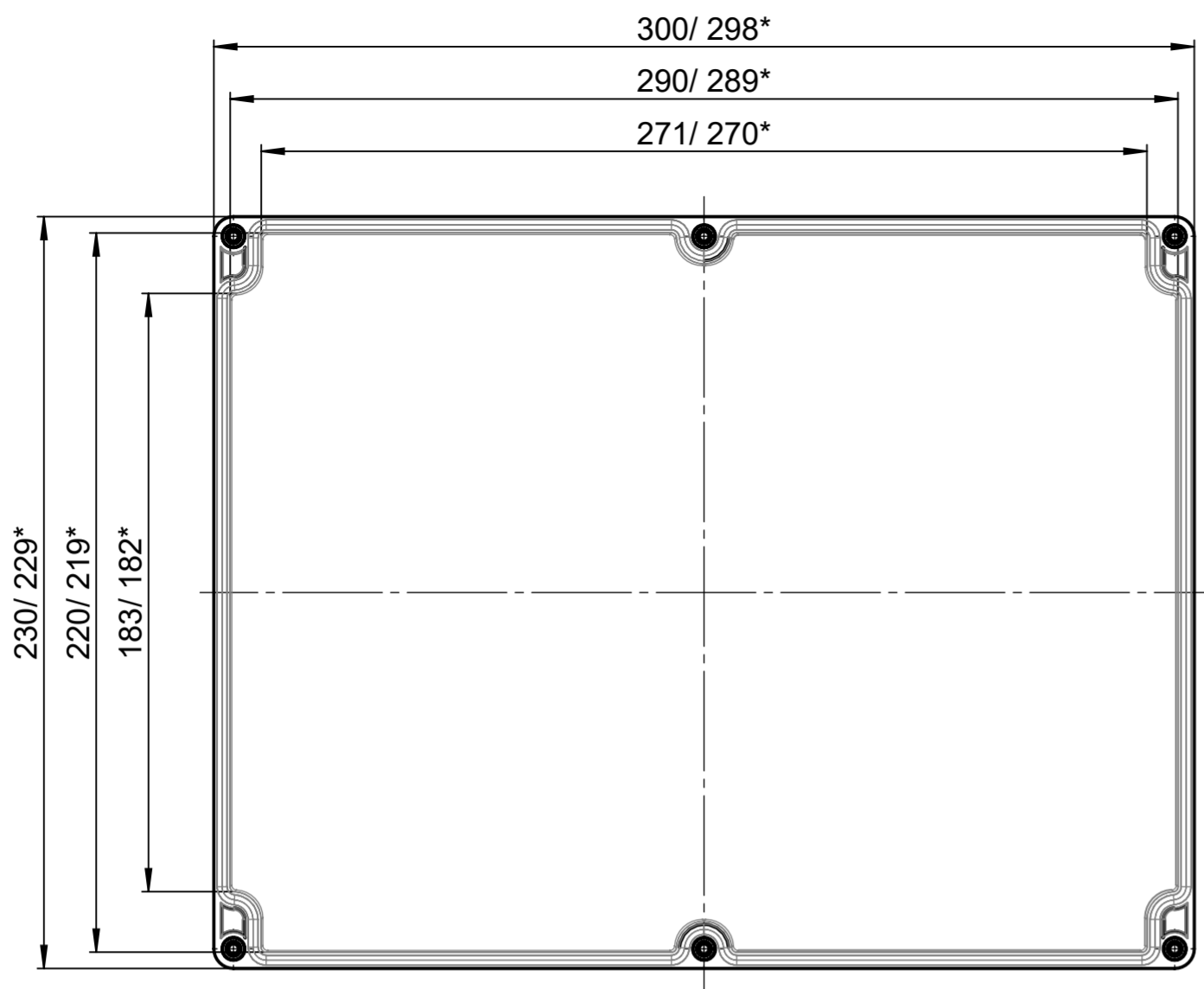
Deckel / Lid
