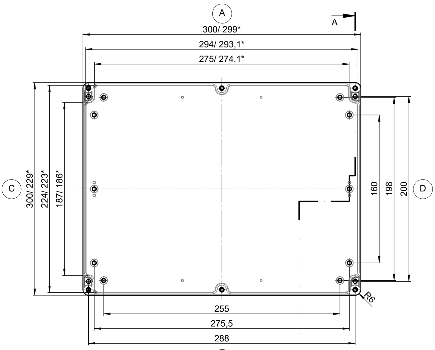
Unterteil / Base
