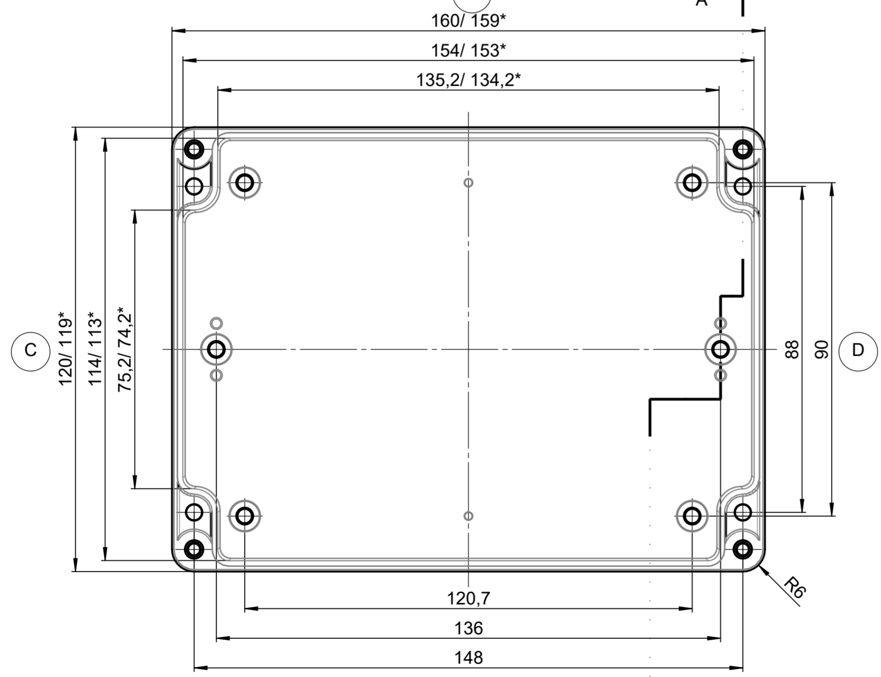
Unterteil / Base
