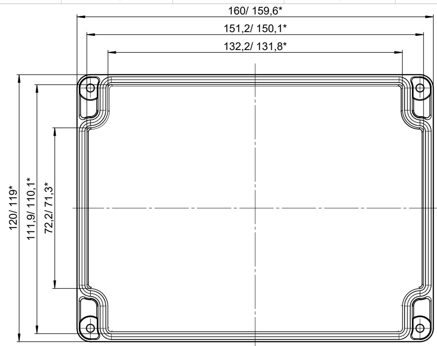
Deckel / Lid
