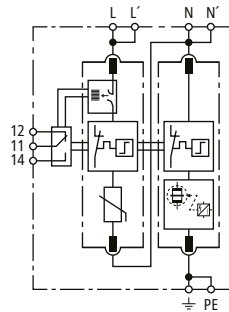
Prinzipschaltbild
