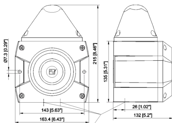
Predisposizione foro M20
