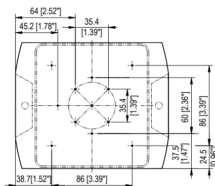
Schema forature interne all'alloggiamento
