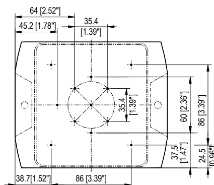
Схема расположения отверстий внутри корпуса
