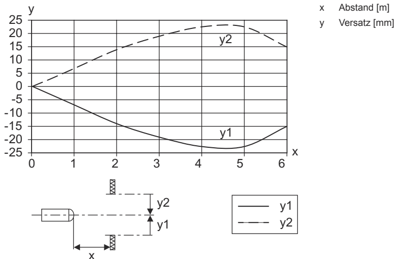
Typ. Funktionsreserve
