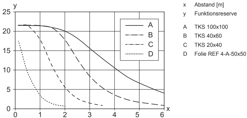
Typ. Funktionsreserve
