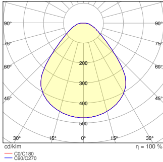
PL CMFT 625 P 30W ML 840 U19 5250lm
