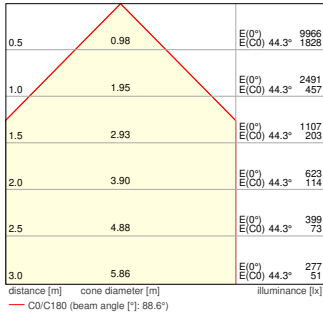
PL CMFT 625 P 30W ML 840 U19 5250lm
