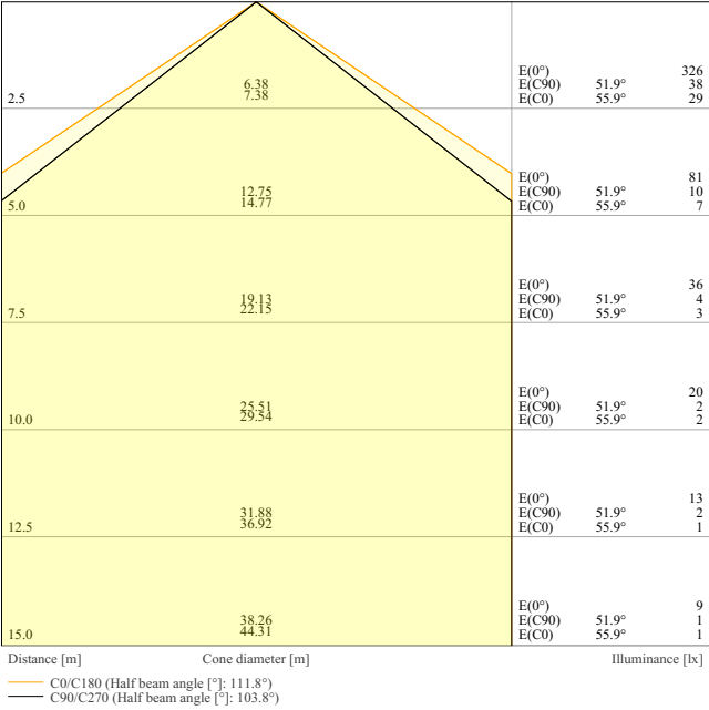
DP 1500 P 36W ML 840 VW IP66
