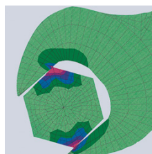
Herkömmlicher Schraubenschlüssel: Kantenpressung führt zu Beschädigung
