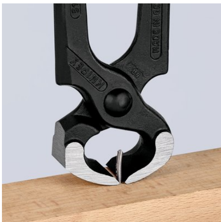
Mehrfachfunktion: Einschlagen und Ziehen von Nägeln
