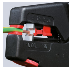
12 40 200: Präzises Abisolieren ohne Beschädigung des Leiters
