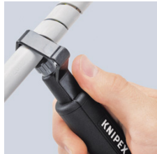
Wendelschnitt
