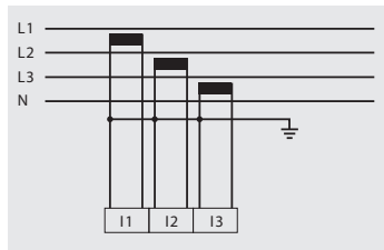
Abb. Messung in einem Dreiphasennetz mit ungleichmäßiger Belastung.
