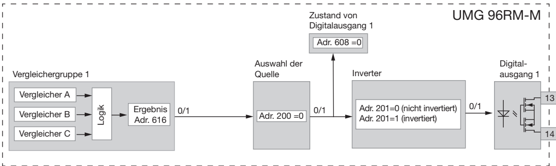
Blockschaltbild: Verwendung des Digitalausganges 1 zur Grenzwertüberwachung.
