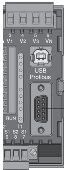
Abb. UMG 96RM-P mit DSub-Buchse für Profibus (Ansicht von hinten).
