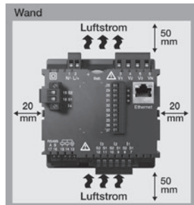
Abb. Einbaulage UMG 96RM-E (Ansicht von hinten)
