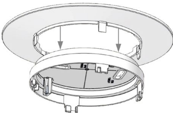
Abb. 1: Blendring aufklipsen
