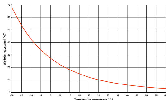
Rys. 7.2: Charakterystyka czujnika NTC-10
