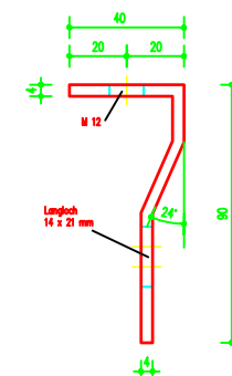
Befestigungswinkel Maßstab 1 : 5
