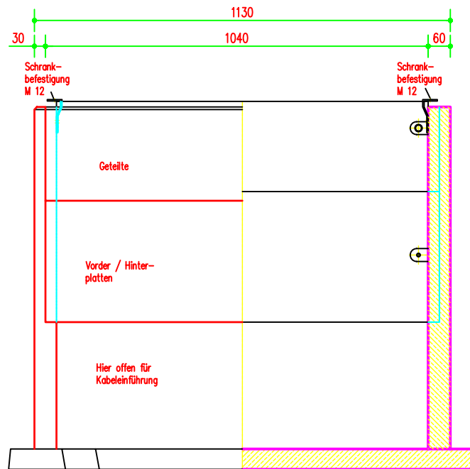
Vorderansicht / Schnitt
