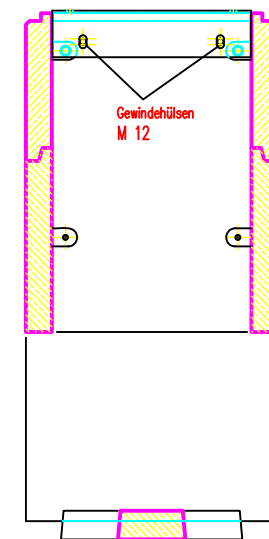
Schnitt
