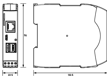
Maßzeichnung Schnittstellen e.Guard-Gateway
