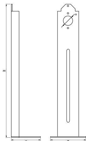
Maßzeichnung Gruppenansicht
