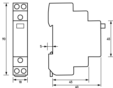
Maßzeichnung Gruppenansicht
