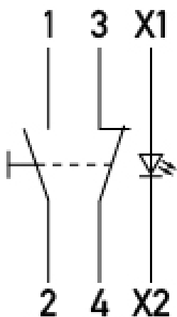
Anschlusschema
