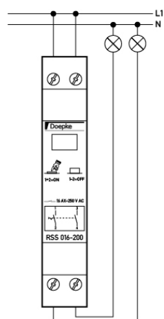
Anschlusschema
