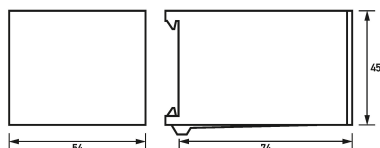
Maßzeichnung Sicherungssteckersätze DSE Do2-50 EI
