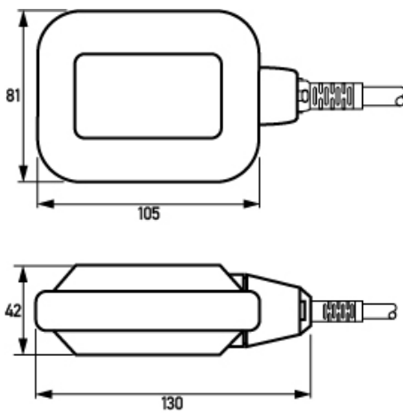
Maßzeichnung Gruppenansicht
