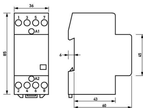
Maßzeichnung Gruppenansicht
