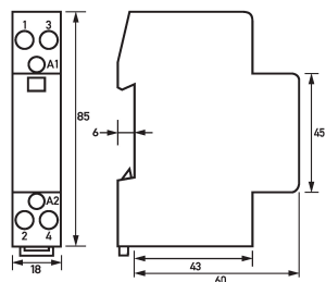
Maßzeichnung Installationsschütze HS 1-024AC/20-11
