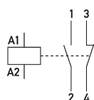
Schaltungsbeispiel Installationsschütze HS 1-024AC/20-11
