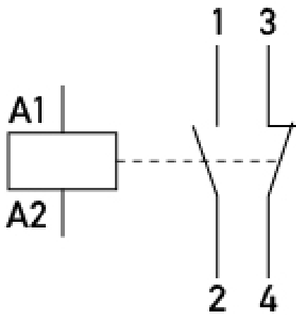
Anschlusschema
