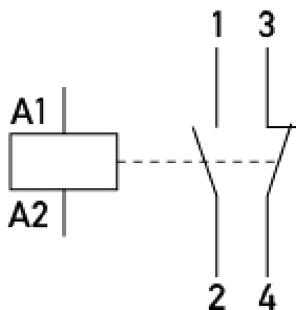
Anschlusschema
