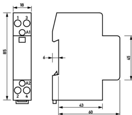
Maßzeichnung Gruppenansicht
