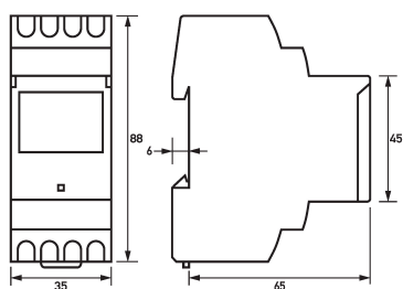
Maßzeichnung Zeitschaltuhren Data Micro 2+
