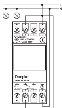
Schaltungsbeispiel Zeitschaltuhren Data Micro 2+
