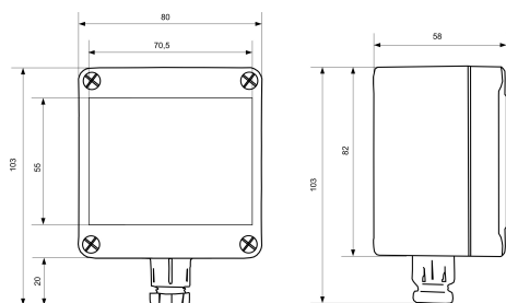
Maßzeichnung Gruppenansicht
