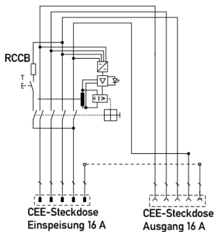
Anschlusschema
