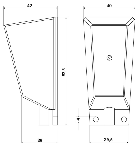
Maßzeichnung Gruppenansicht
