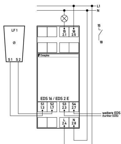
Anschlussschema
