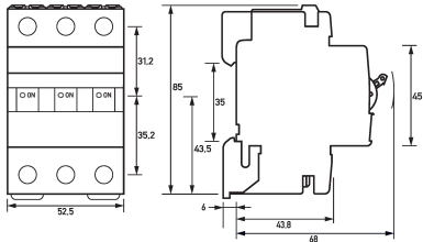
Maßzeichnung Gruppenansicht
