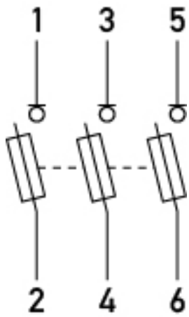
Anschlusschema
