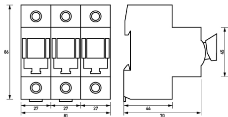
Maßzeichnung Gruppenansicht
