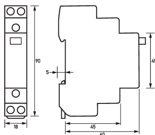
Maßzeichnung Stromstoßschalter (Fernschalter) RS 230-200
