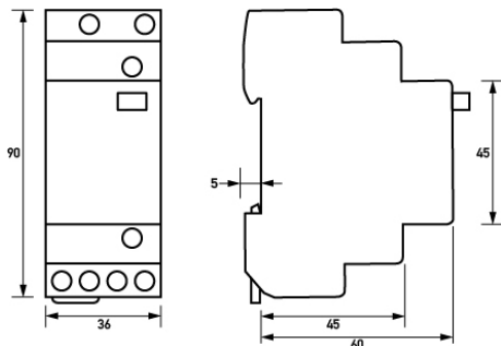
Maßzeichnung Gruppenansicht
