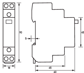
Maßzeichnung Installationsrelais RI 024-110 DC
