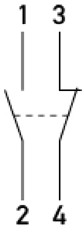
Anschlusschema
