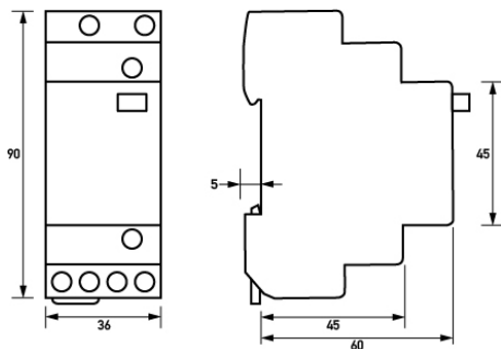
Maßzeichnung Gruppenansicht
