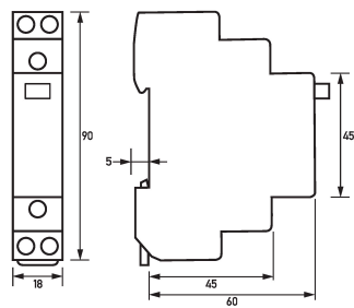
Maßzeichnung Installationsrelais RI 012-001
