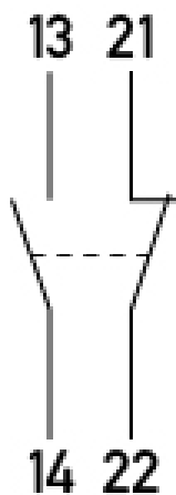
Anschlussschema
