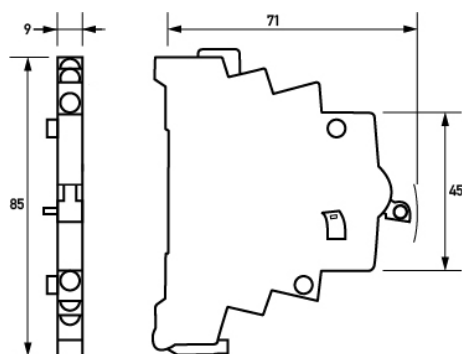
Maßzeichnung Gruppenansicht
