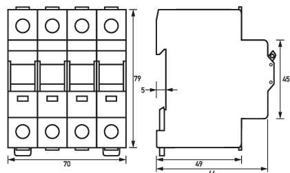
Maßzeichnung Lasttrennschalter RH 063-400
