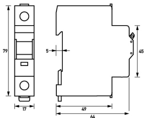
Maßzeichnung Gruppenansicht
