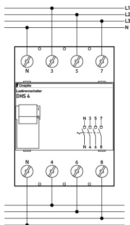
Anschlusschema
